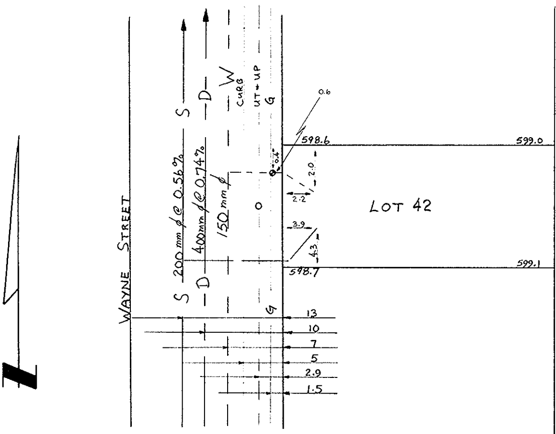
SITE PLAN N.T.S.
