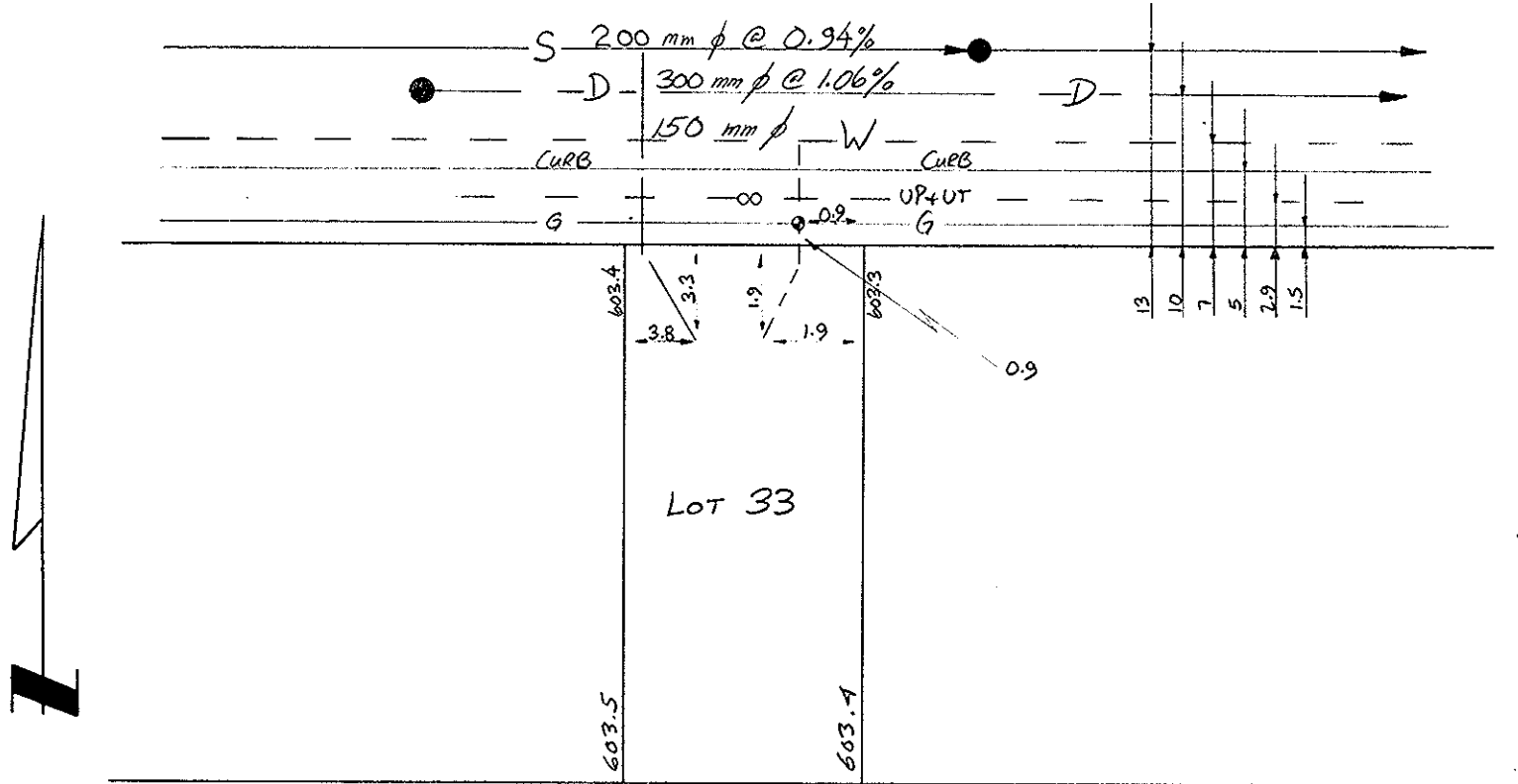
GRACE CRES SITE PLAN N.T.S.
