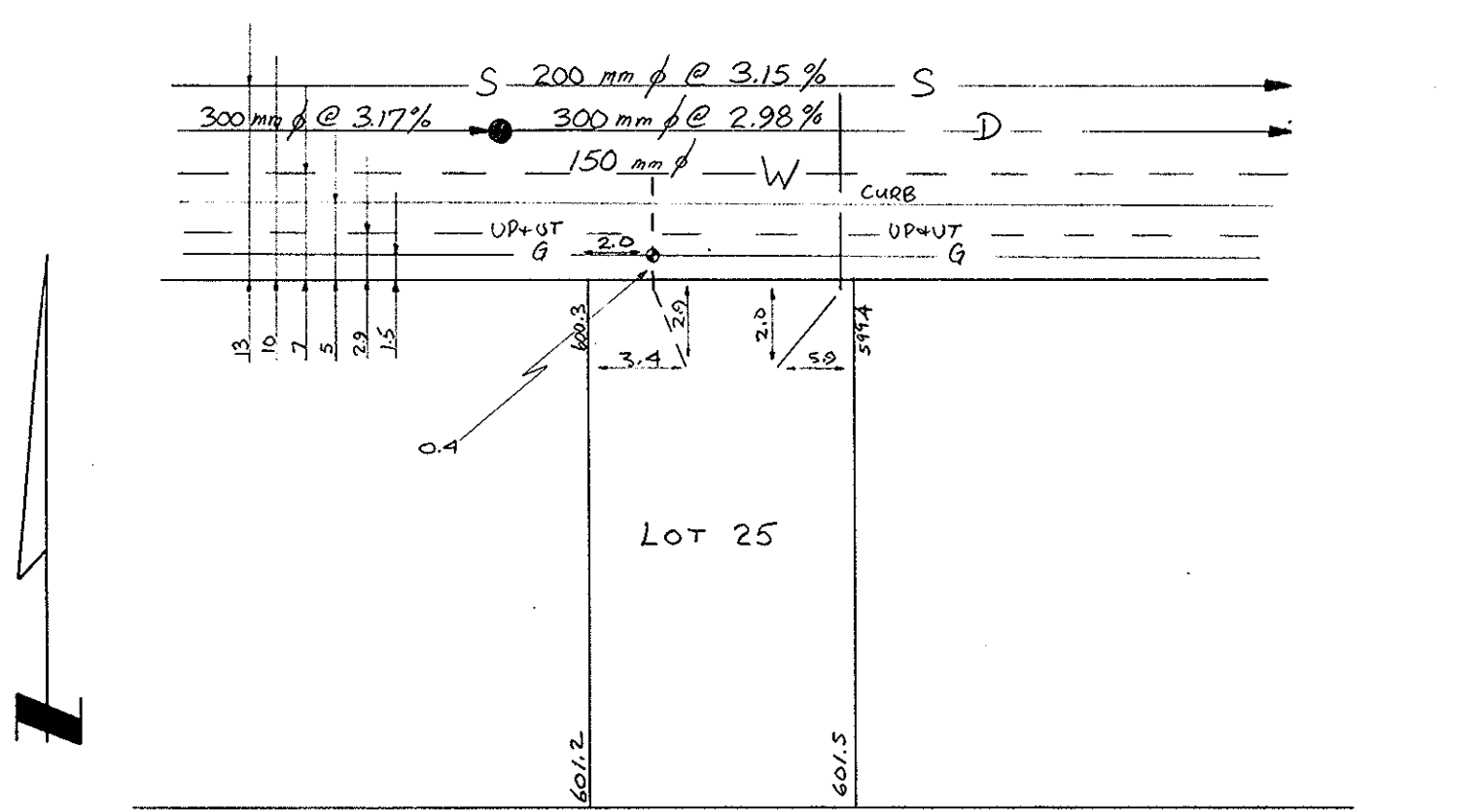
SHANE CRES. SITE PLAN N.T.S.
