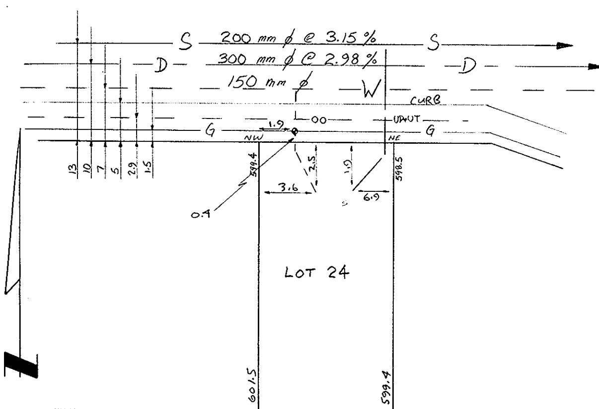
SHANE CRES. SITE PLAN N.T.S.
