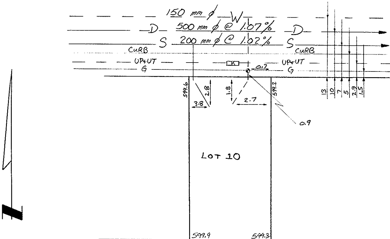
SITE PLAN N.T.S. SHANE CRES.
