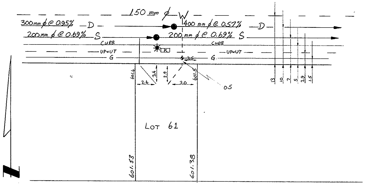
SITE PLAN N.T.S. GRACE CRES.
