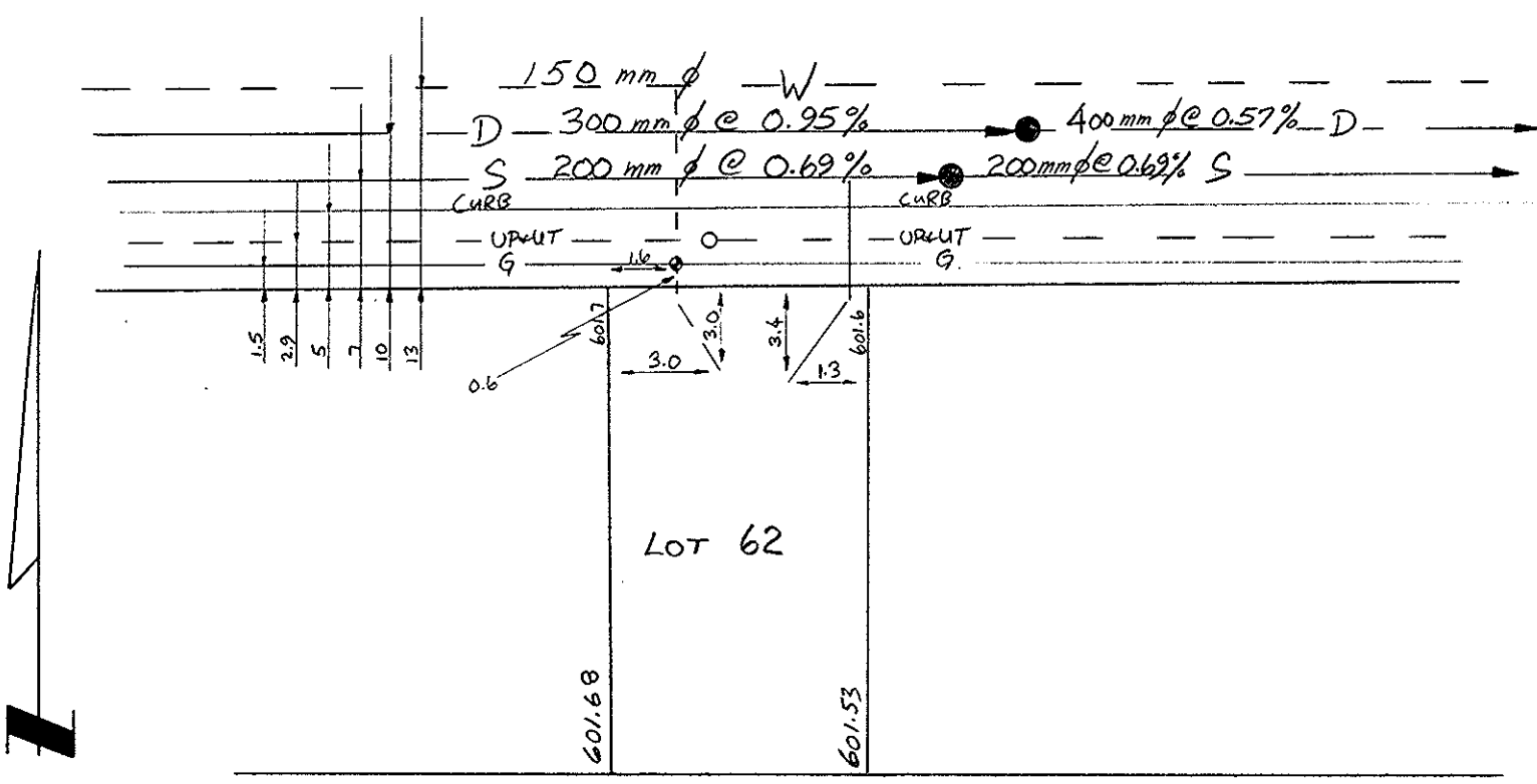
SITE PLAN N.T.S. GRACE CRES.
