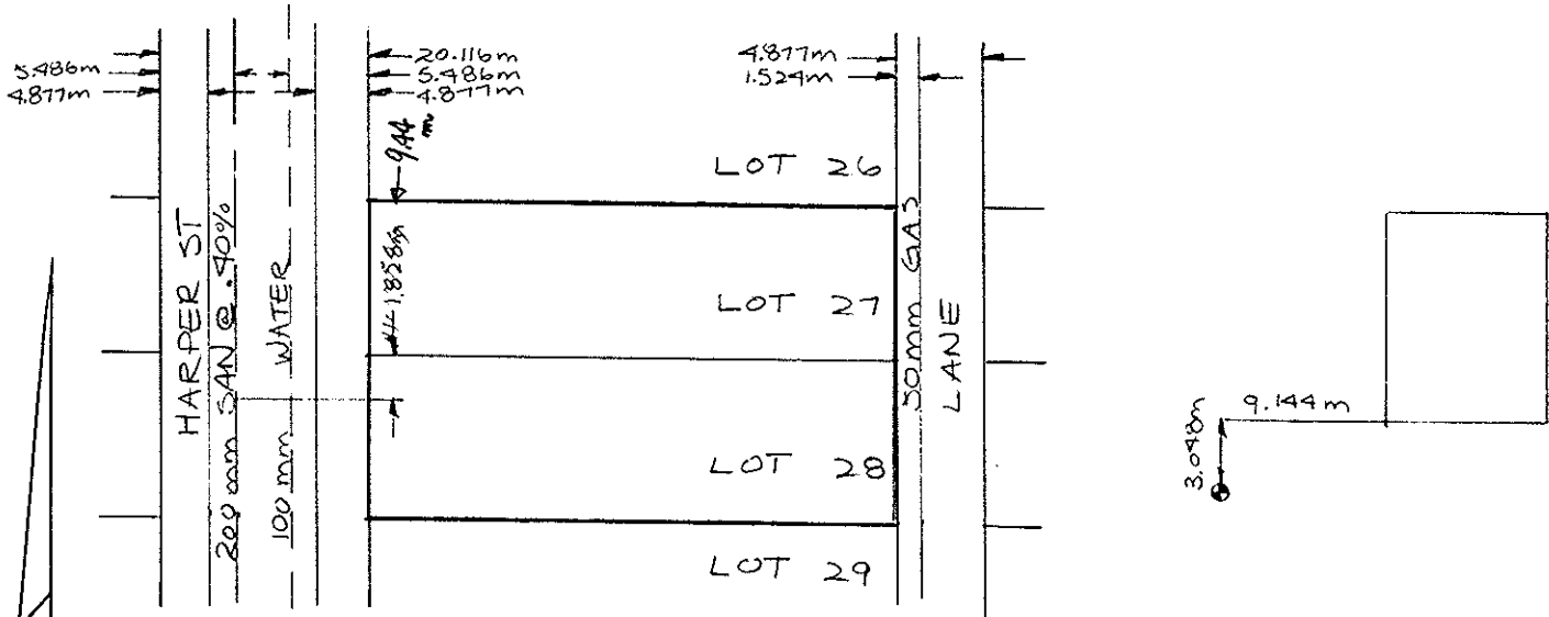
SITE PLAN N.T.S.
