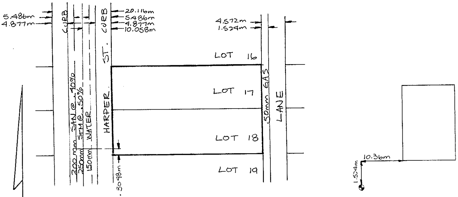
SITE PLAN N.T.S.
