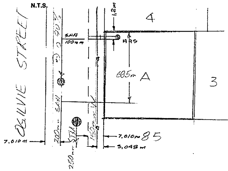
SITE PLAN N.T.S.
