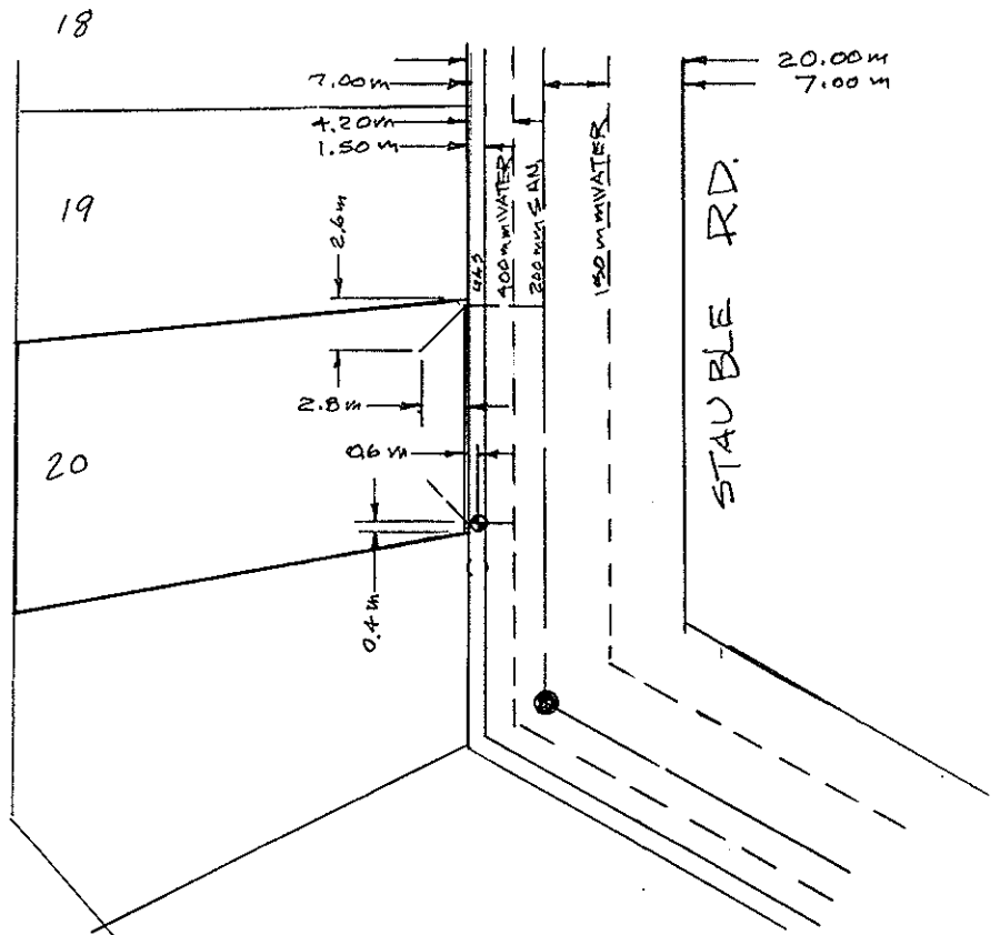
SITE PLAN N.T.S.
