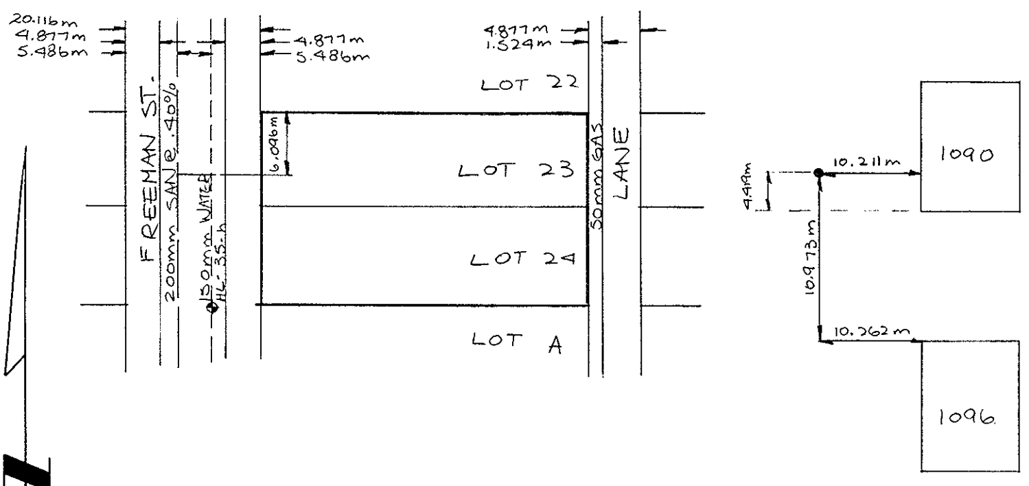
SITE PLAN N.T.S.
