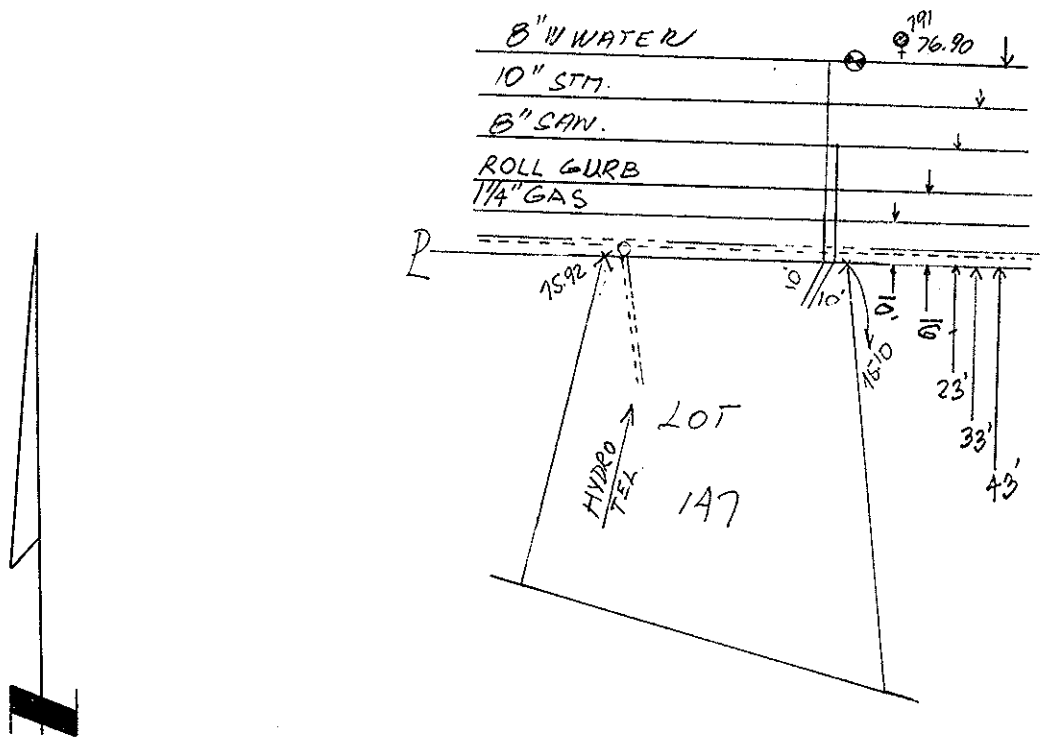
SITE PLAN N.T.S. GUEST CRESCENT
