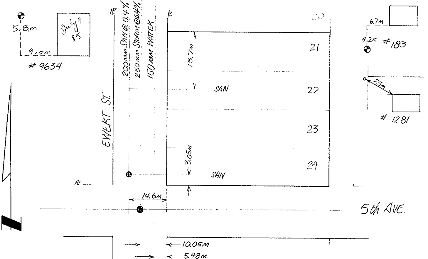
SITE PLAN N.T.S.
