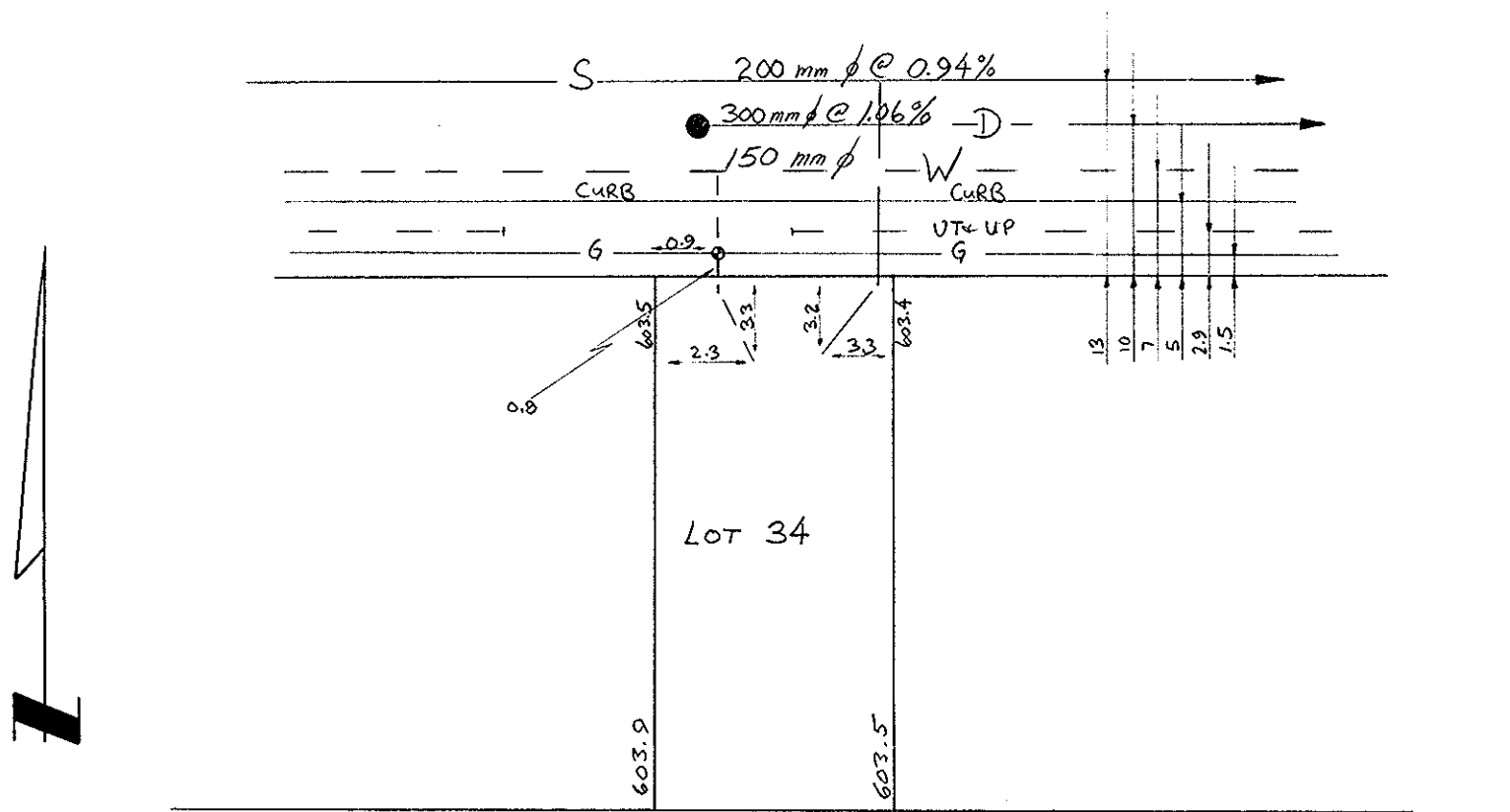
SITE PLAN N.T.S. GRACE CRES
