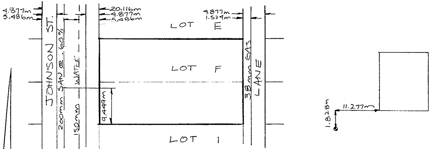
SITE PLAN N.T.S.
