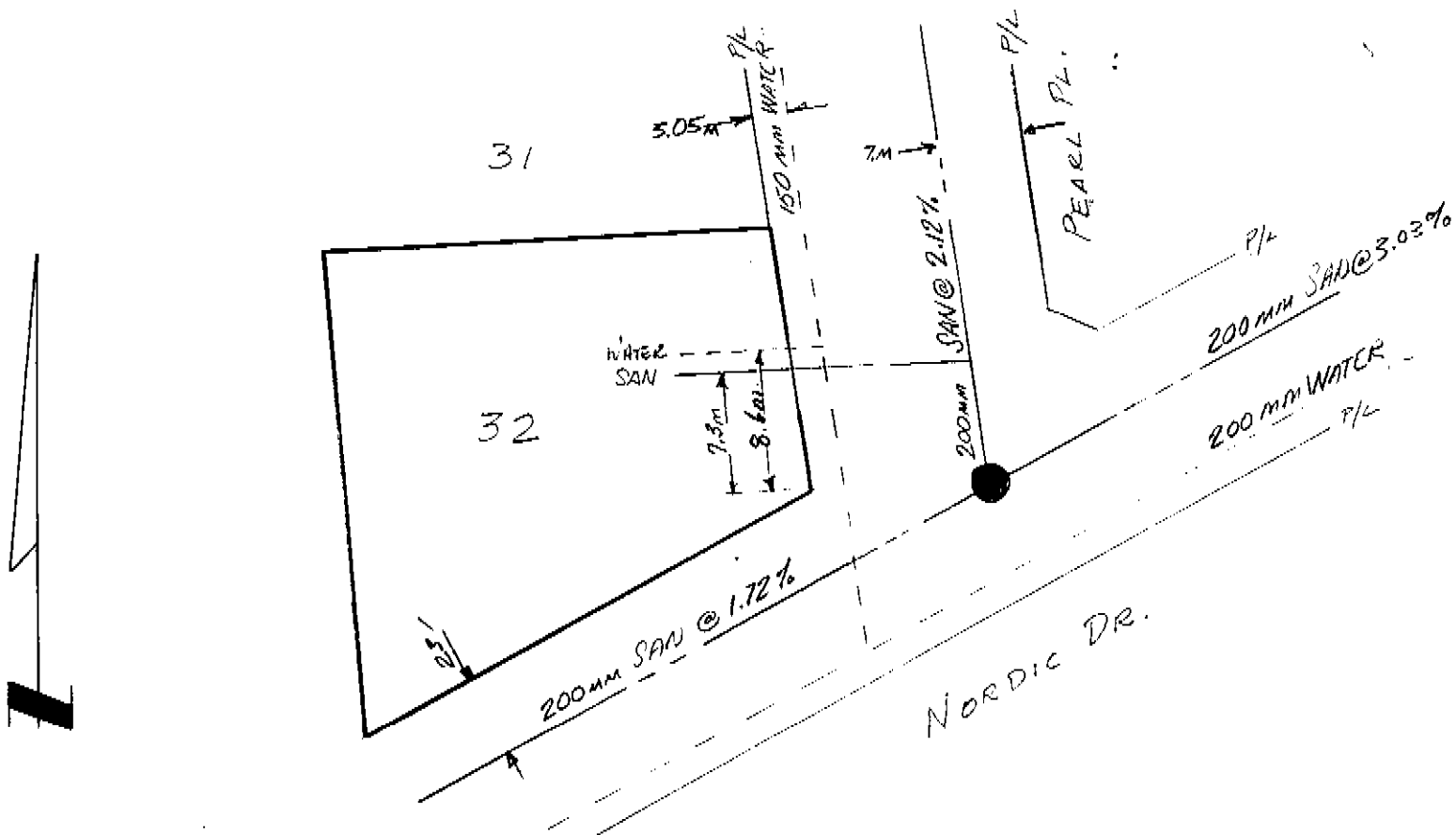
SITE PLAN N.T.S.
