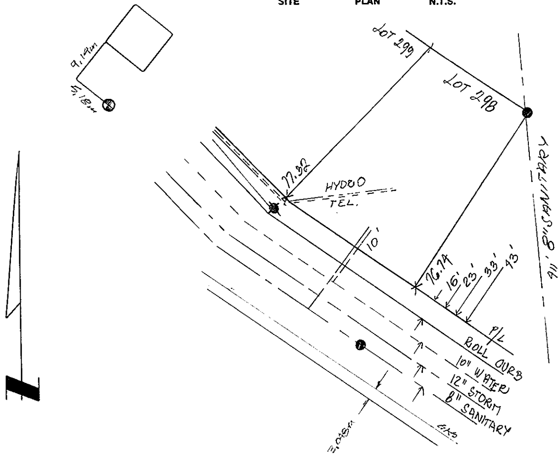
SITE PLAN N.T.S.
