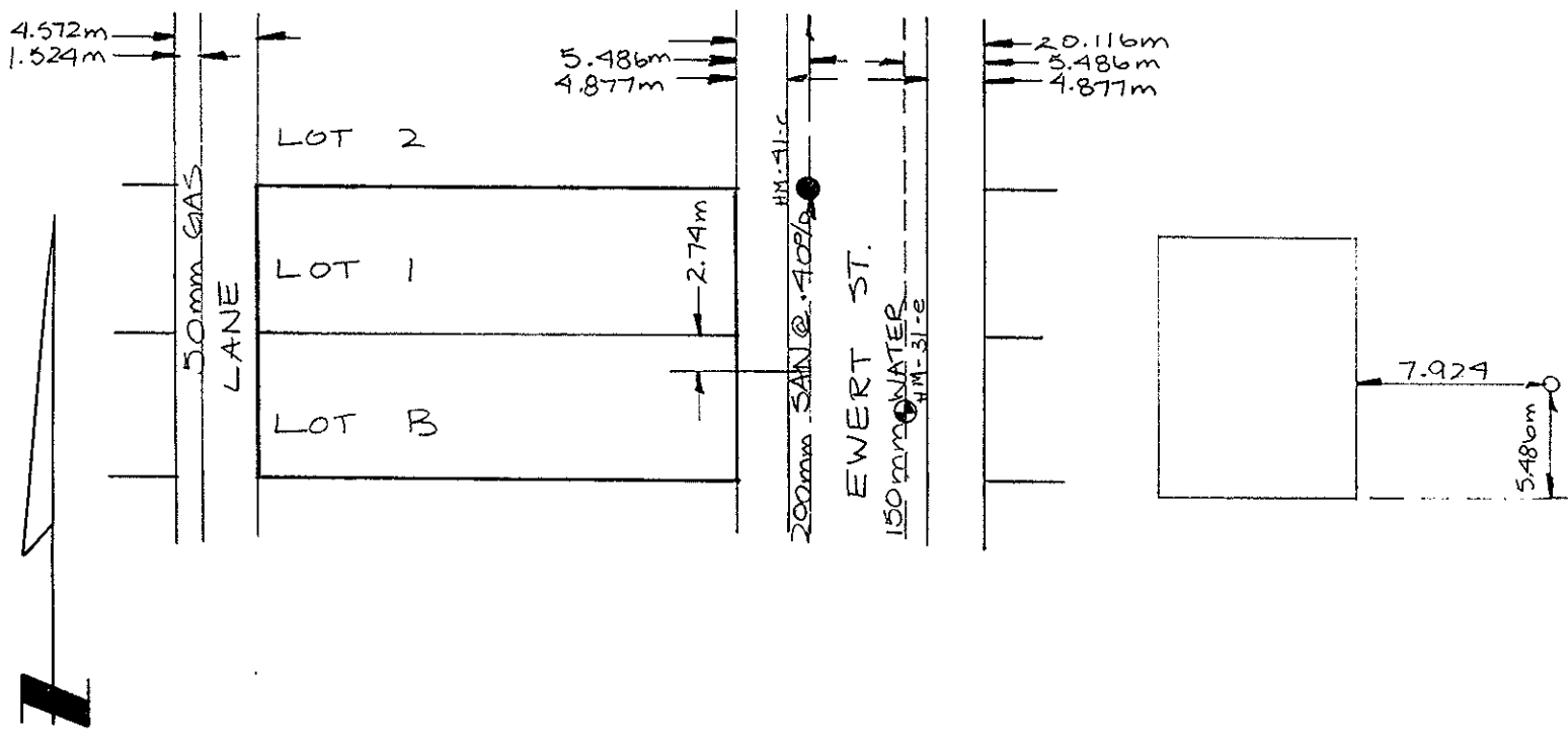
SITE PLAN N.T.S.
